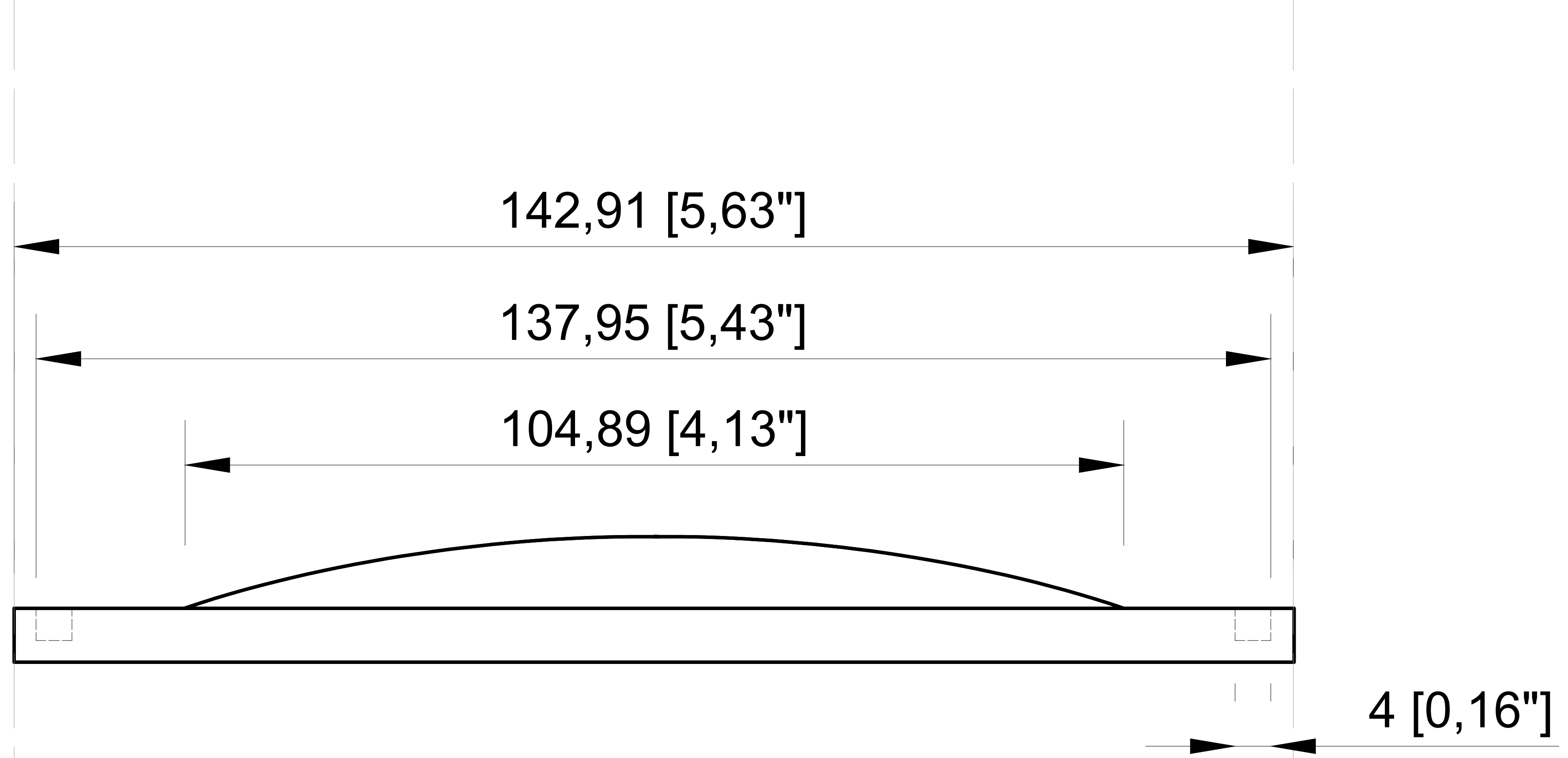
Vista lateral
